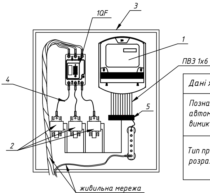
Монтажна схема
